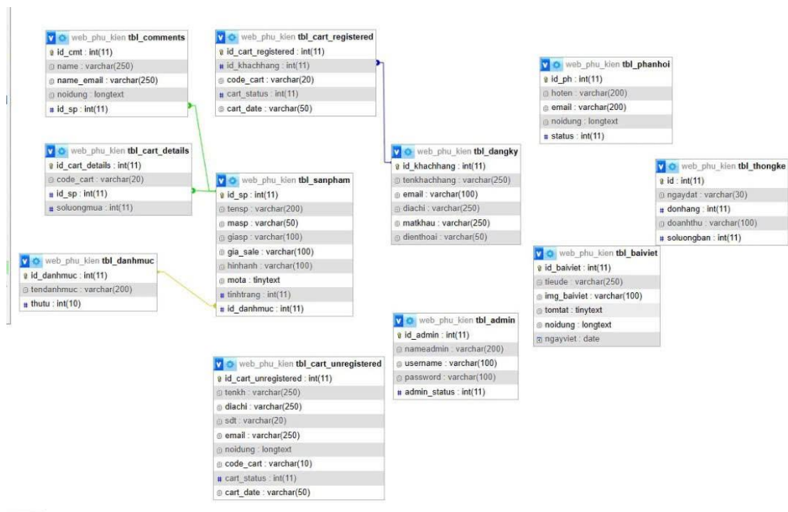
Hình 3.2 Mô hình dữ liệu
