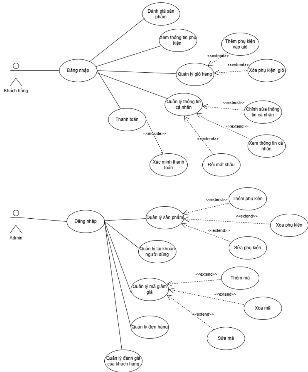
Hình 3.3 Mô hình use case
